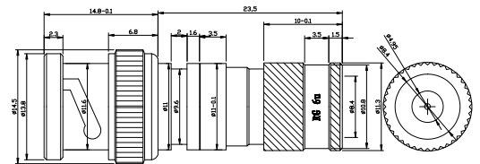
Spina BNC a pressione per CAVI RG6U
