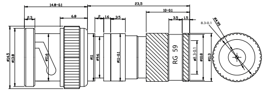
Spina BNC a pressione per CAVI RG59
