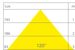
DISTRIBUZIONE LUCE 30W
