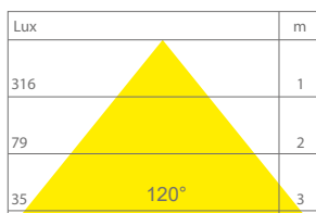
DISTRIBUZIONE LUCE 12W
