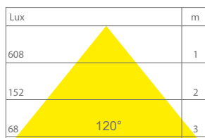
DISTRIBUZIONE LUCE 25W
